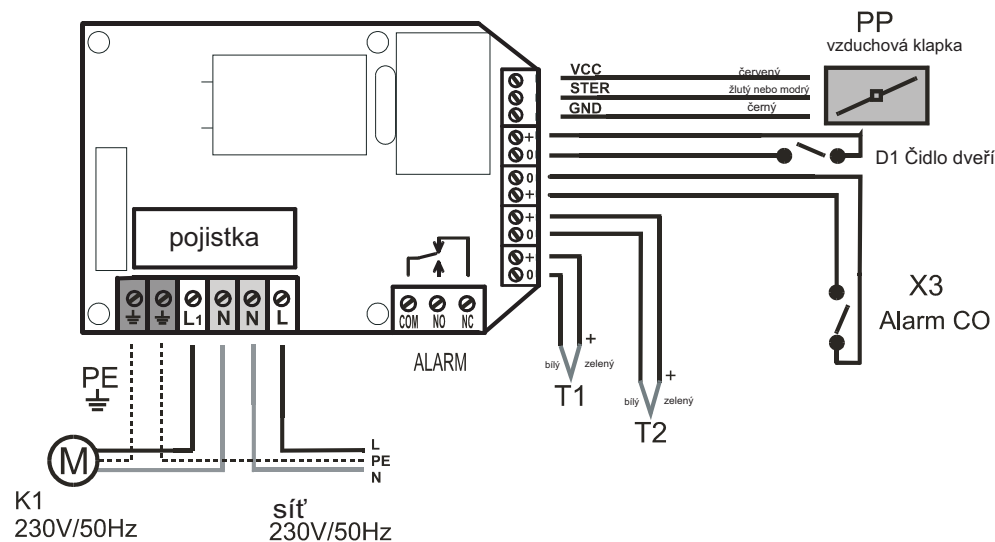
Obr. 3 Schéma elektroinstalace
